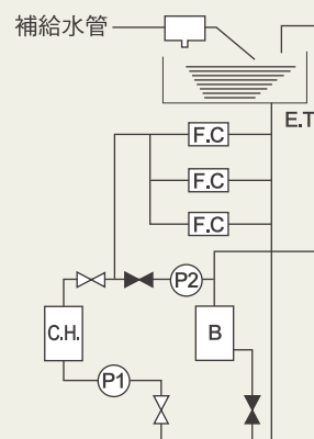
〈冰水機配管圖例〉
